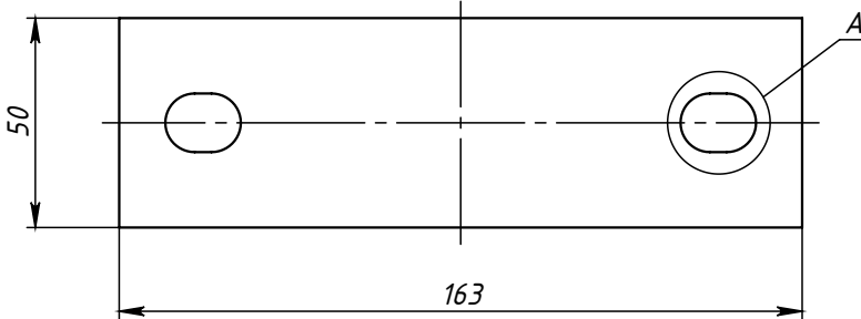
Поз.1 (Полухомут) развертка
