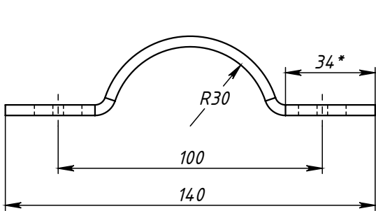
Поз.1 (Полухомут)
